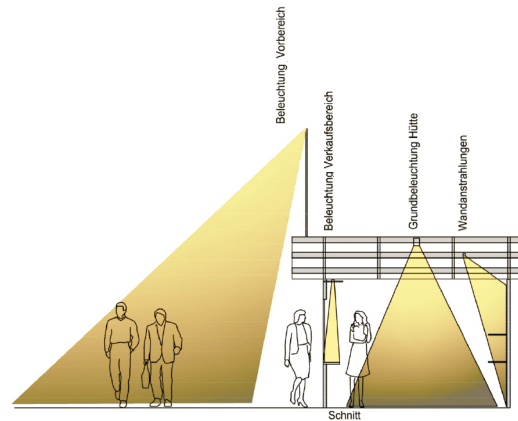
Schnitt
